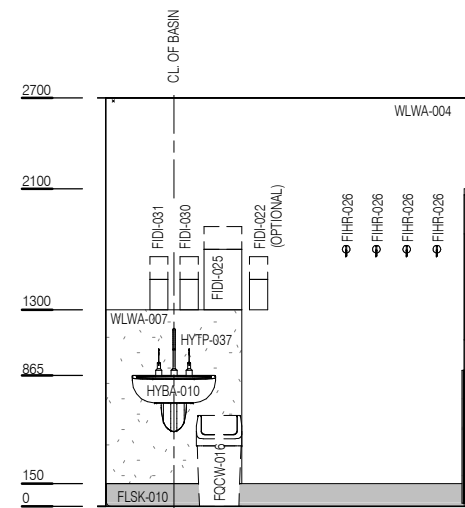
ELEVATION 1
