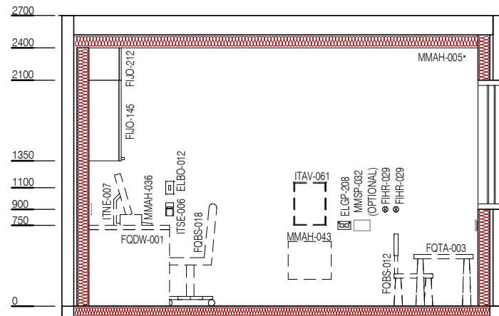
ELEVATION 2
