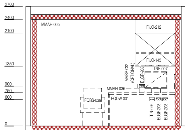
ELEVATION 1
