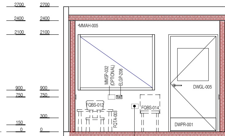
ELEVATION 3
