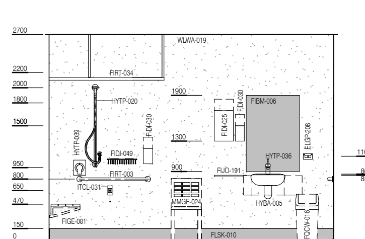
ELEVATION 3
