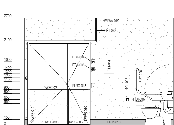
ELEVATION 1
