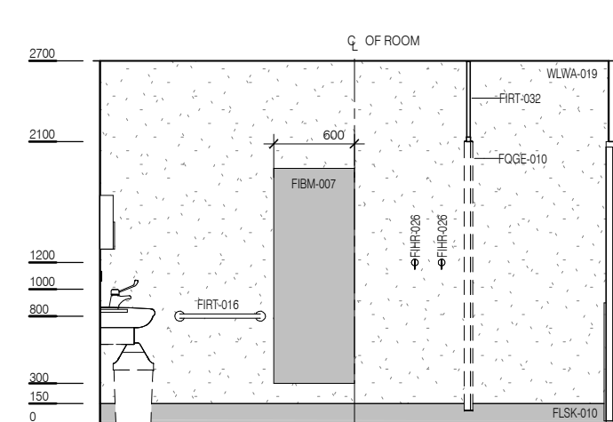
ELEVATION 4
