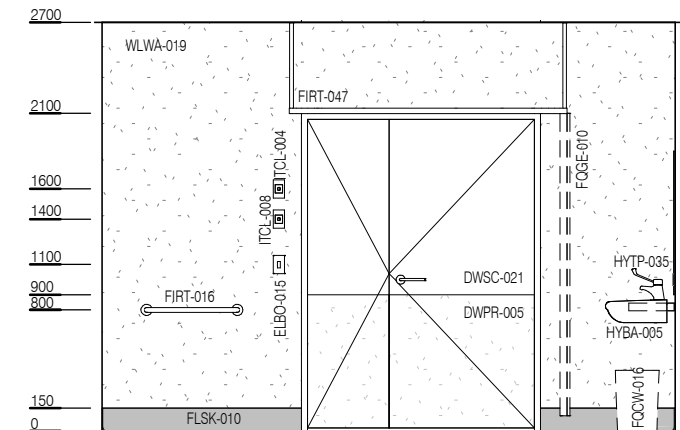
ELEVATION 4
