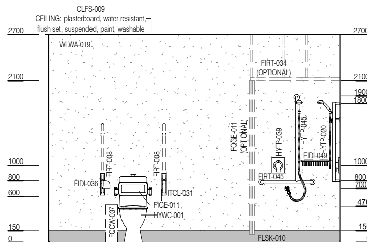
ELEVATION 2
