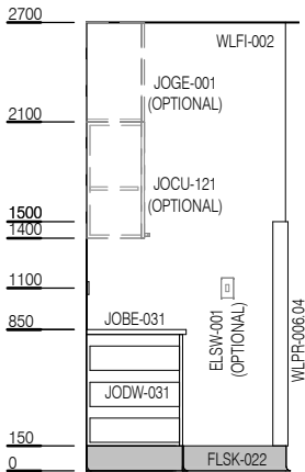
ELEVATION 3
