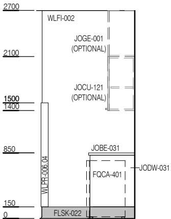
ELEVATION 1
