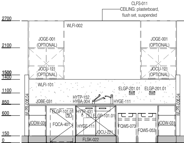
ELEVATION 2
