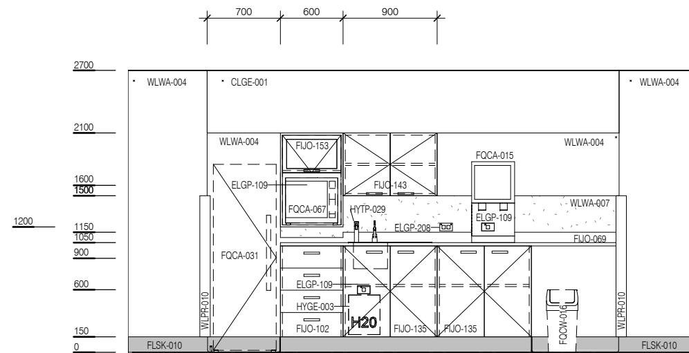
ELEVATION 2
