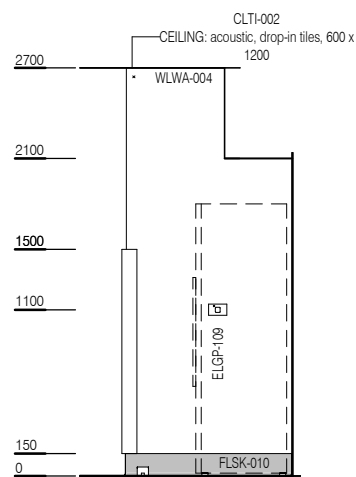
ELEVATION 1
