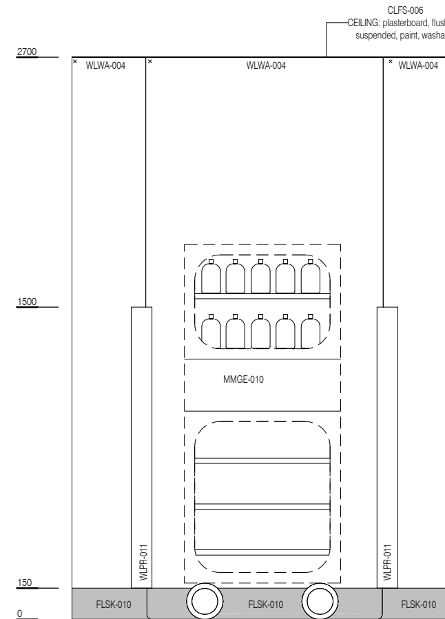
ELEVATION 2
