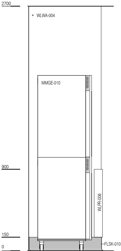
ELEVATION 3
