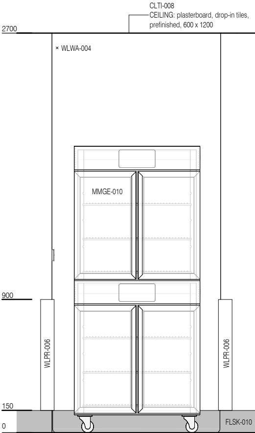
ELEVATION 2
