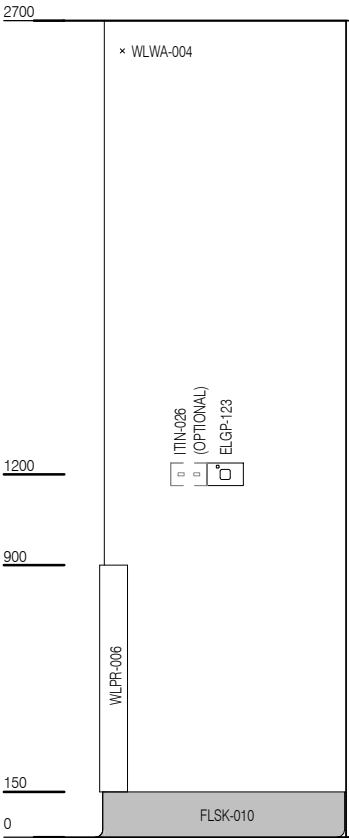
ELEVATION 1
