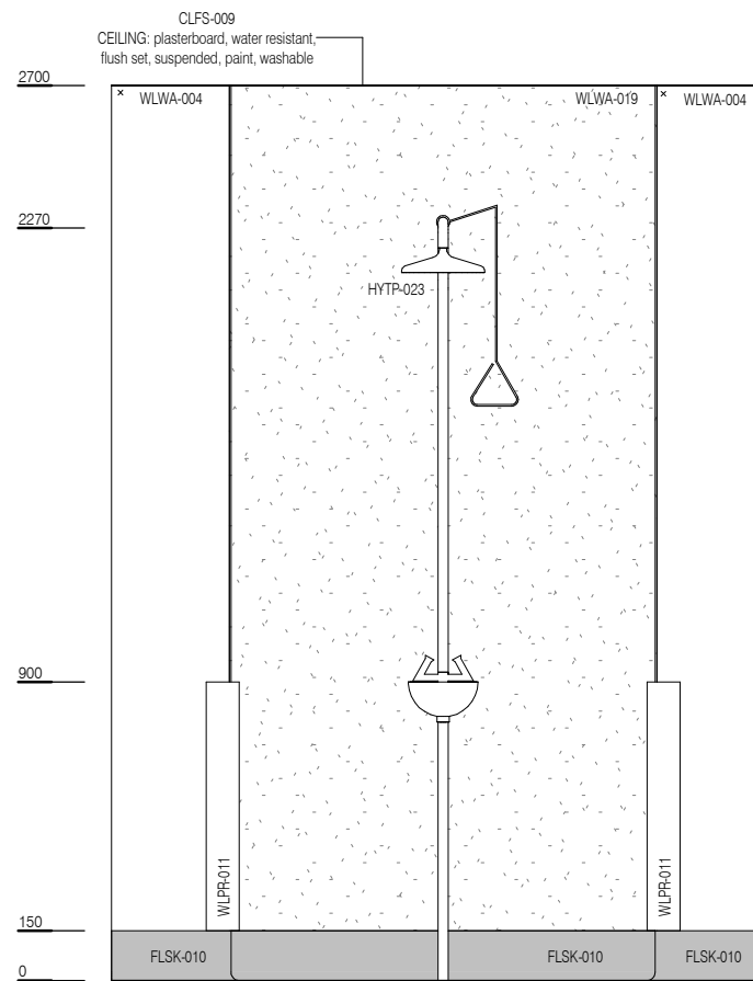
ELEVATION 1
