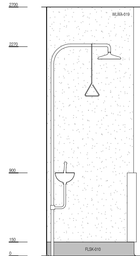
ELEVATION 2
