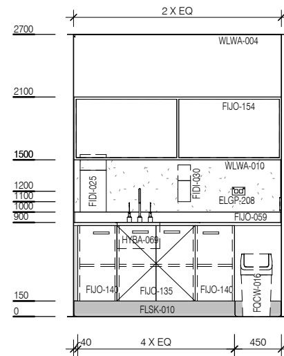
ELEVATION 1
