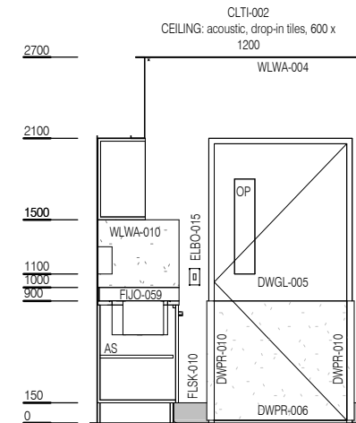
ELEVATION 2
