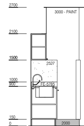
ELEVATION 3
