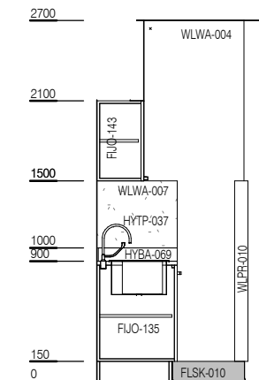
ELEVATION 3
