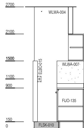
ELEVATION 1
