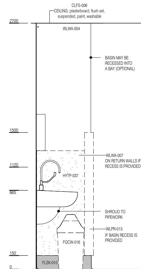
ELEVATION 2
