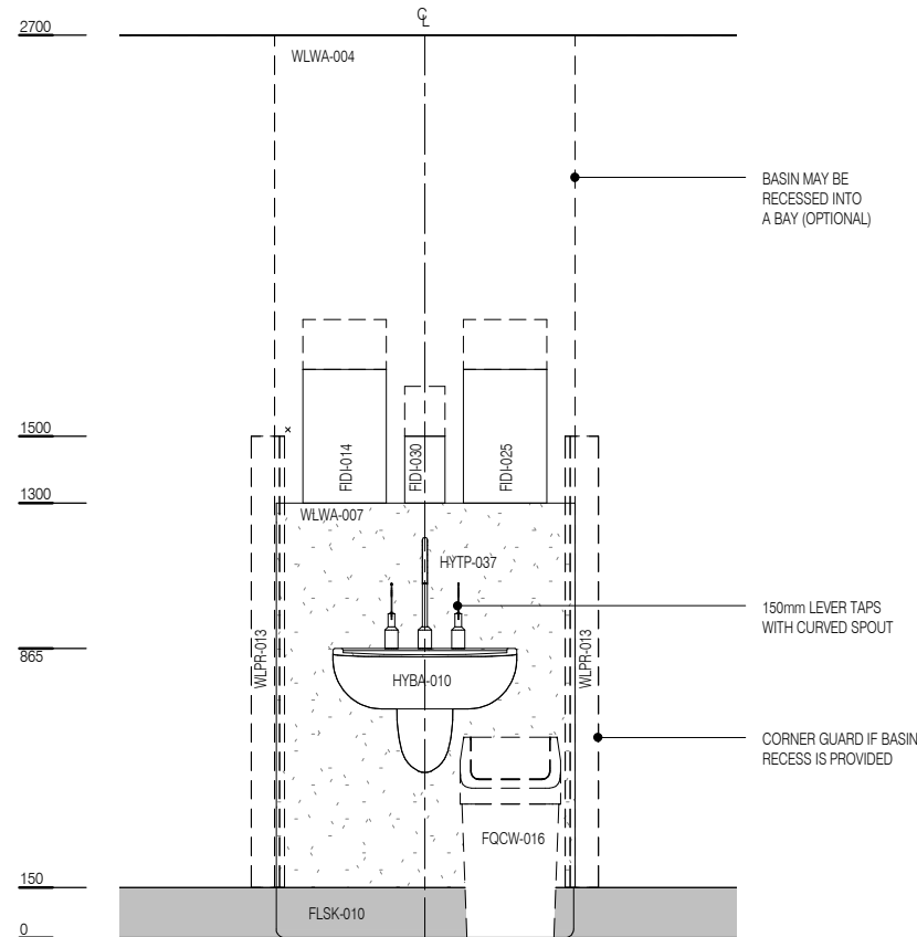
ELEVATION 1
