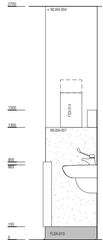
ELEVATION 3
