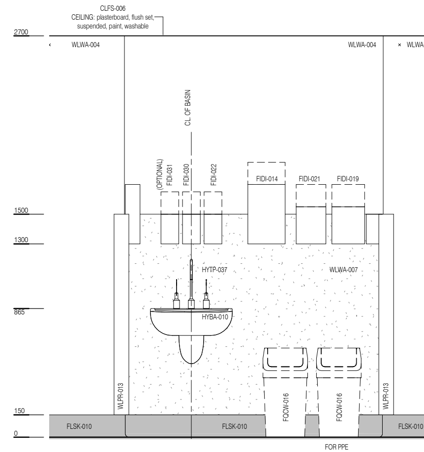
ELEVATION 2
