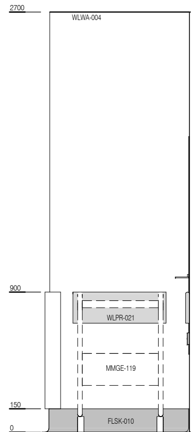
ELEVATION 1
