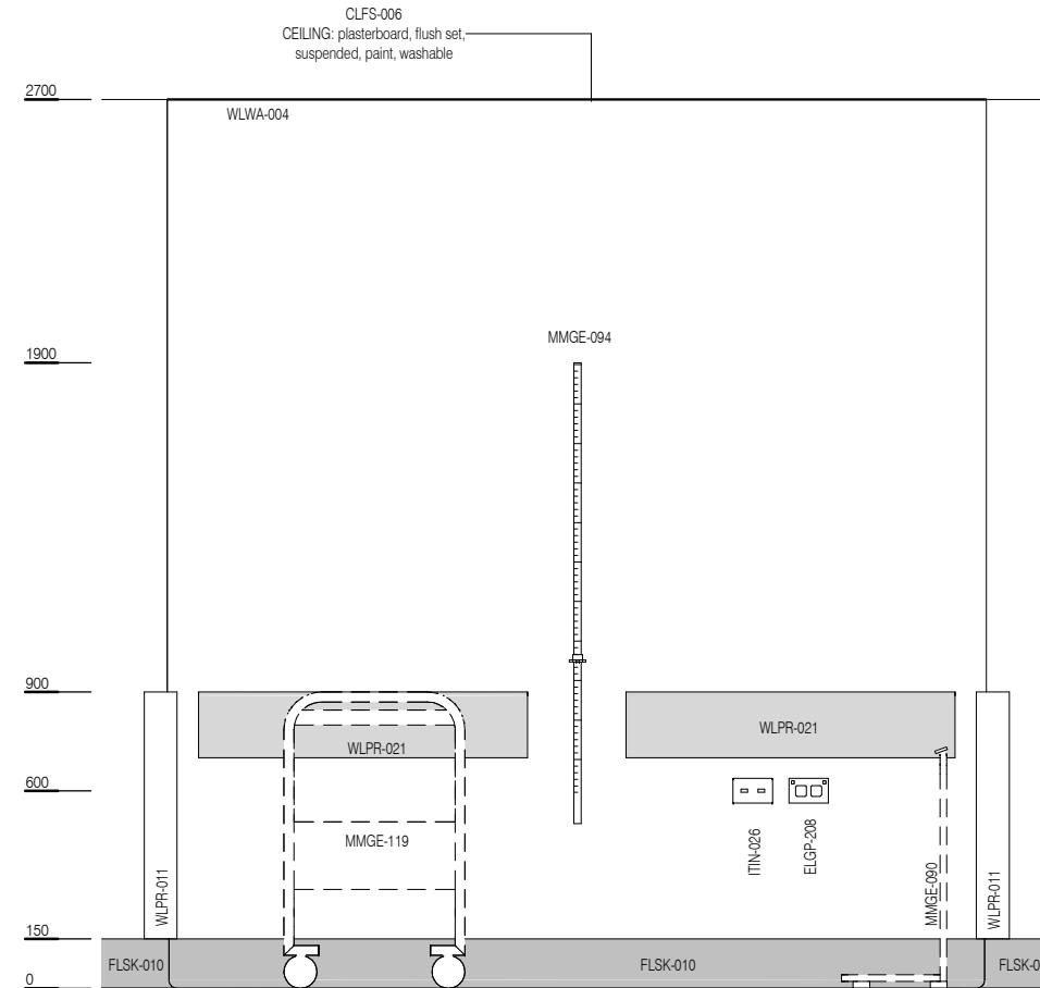
ELEVATION 2
