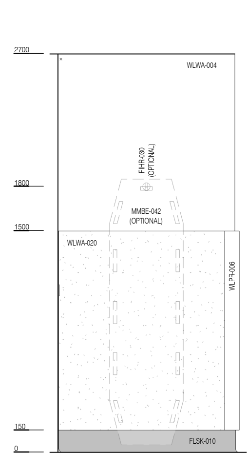
ELEVATION 3
