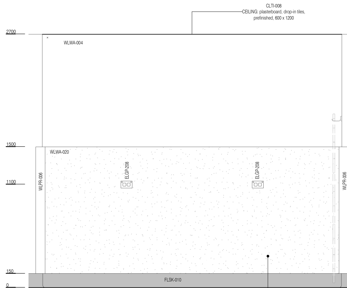
ELEVATION 2
