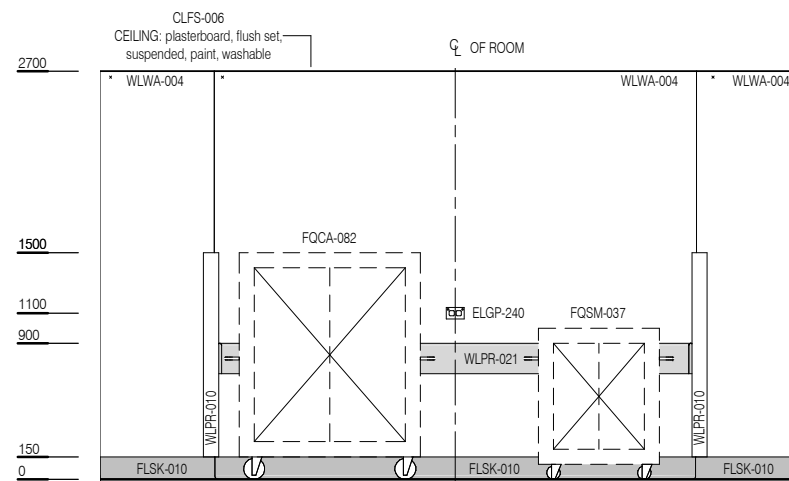
ELEVATION 2
