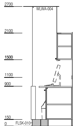
ELEVATION 1
