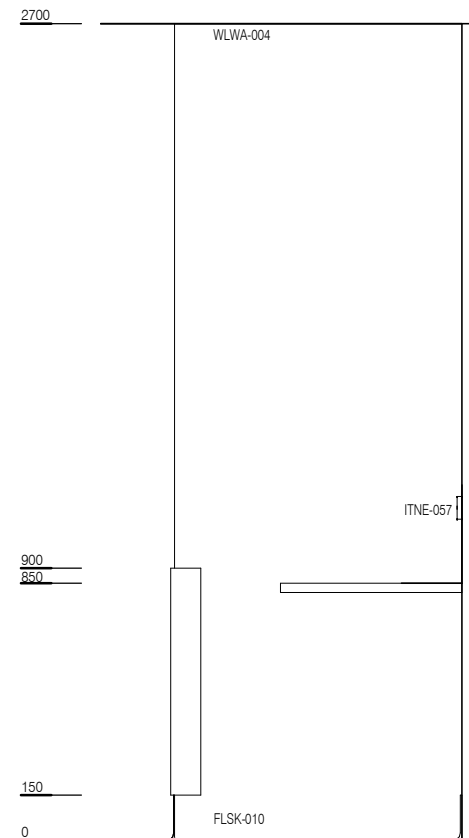
ELEVATION 1
