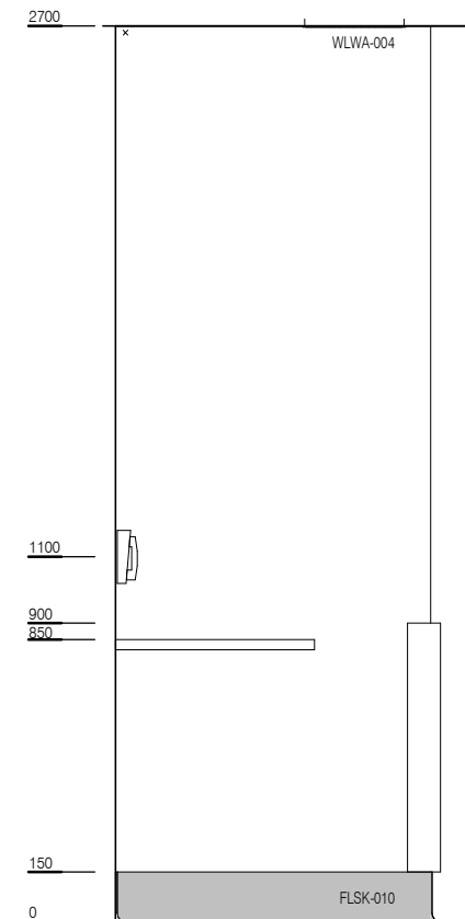
ELEVATION 3
