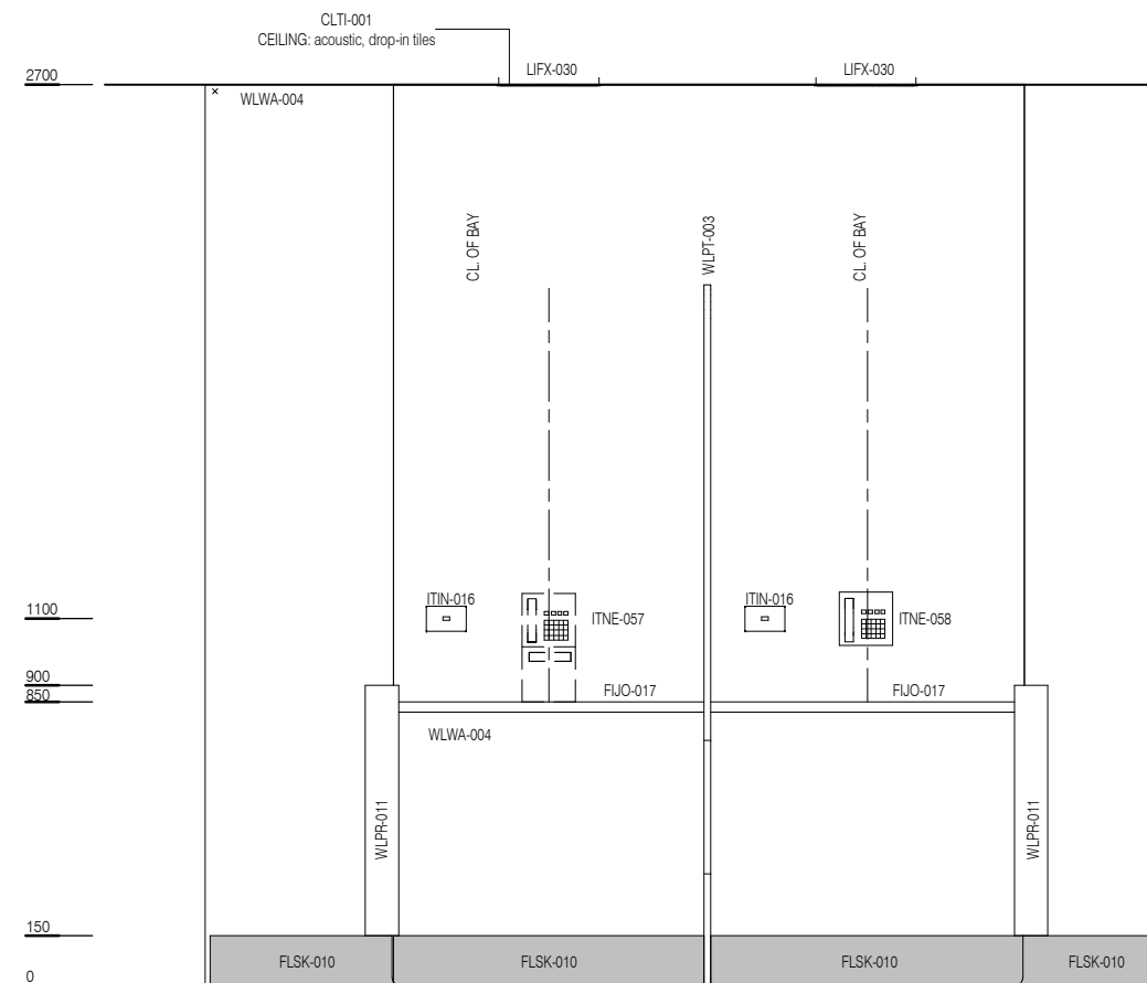
ELEVATION 2
