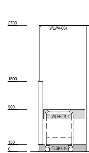
ELEVATION 1
