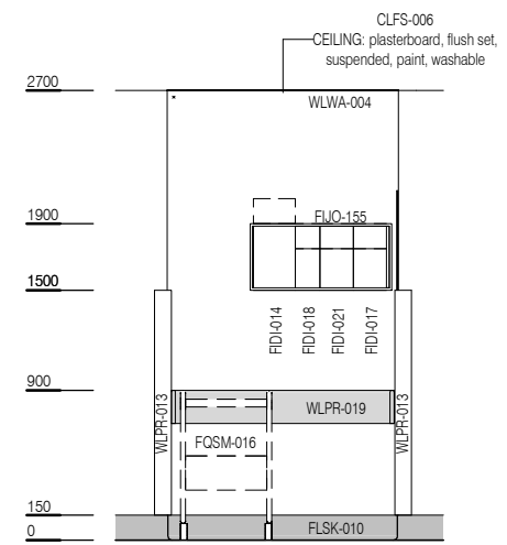
ELEVATION 2
