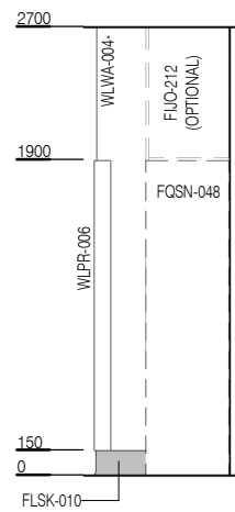
ELEVATION 1
