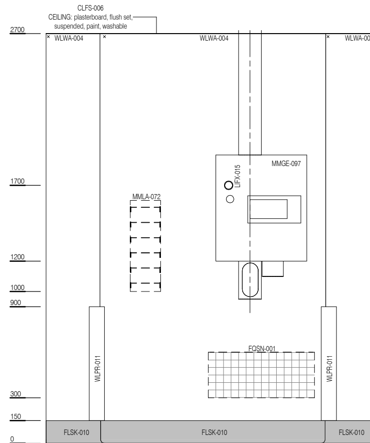
ELEVATION 2
