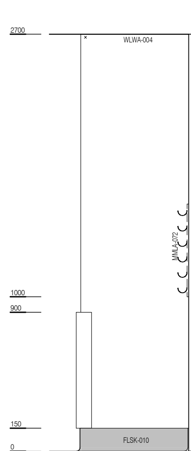
ELEVATION 1
