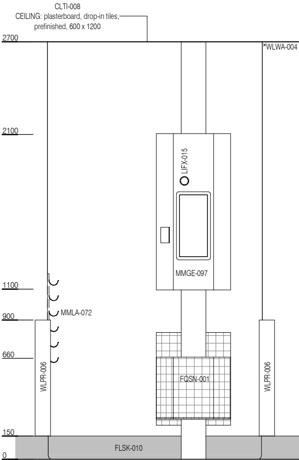
ELEVATION 2
