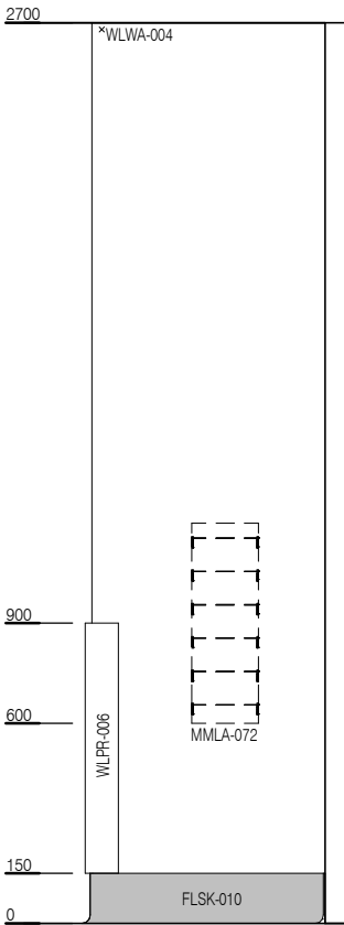
ELEVATION 1
