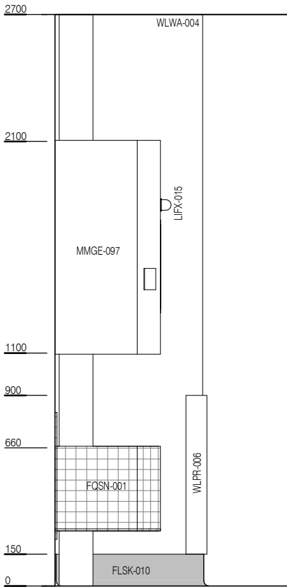
ELEVATION 3
