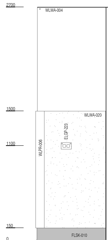
ELEVATION 1
