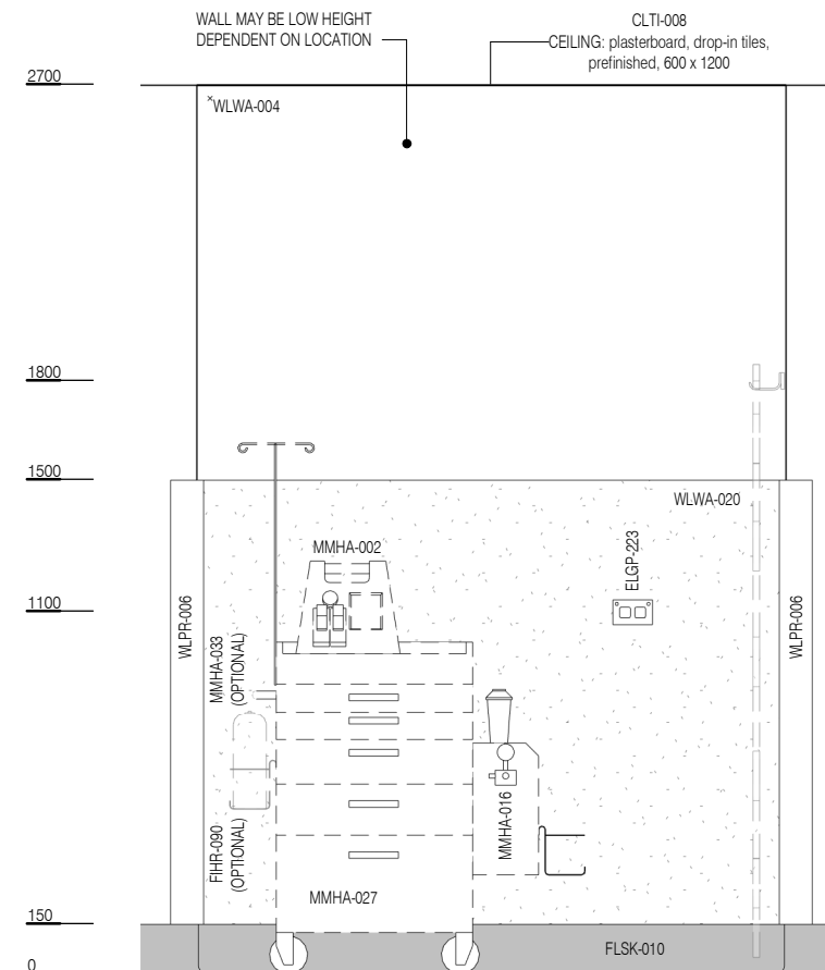
ELEVATION 2
