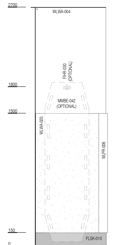
ELEVATION 3
