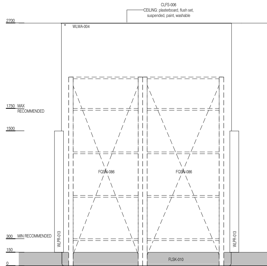
ELEVATION 2
