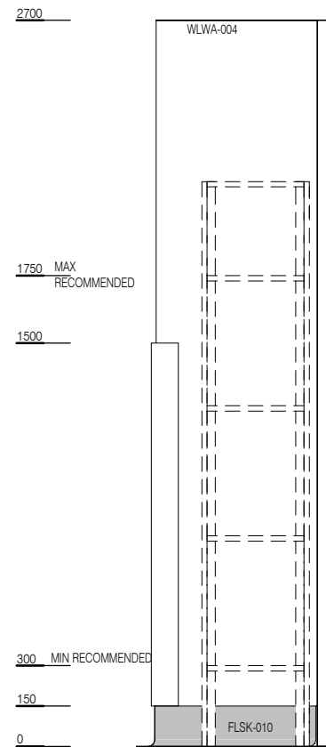
ELEVATION 1
