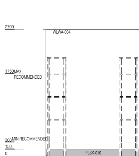
ELEVATION 1
