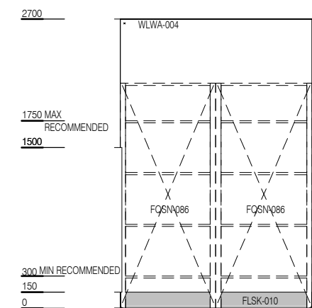
ELEVATION 4
