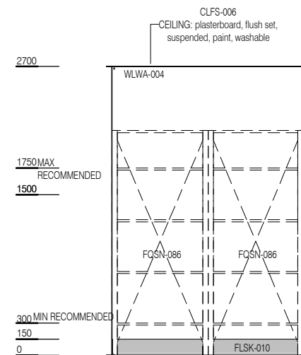
ELEVATION 2
