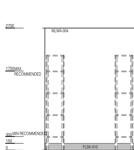
ELEVATION 1
