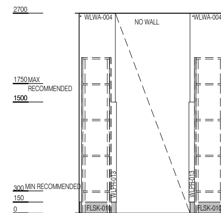
ELEVATION 3
