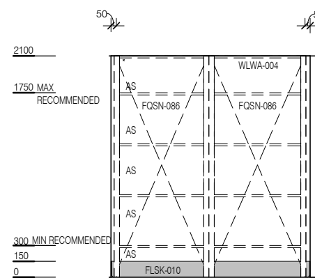
ELEVATION 2
