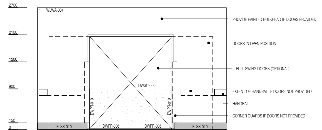
ELEVATION 3
