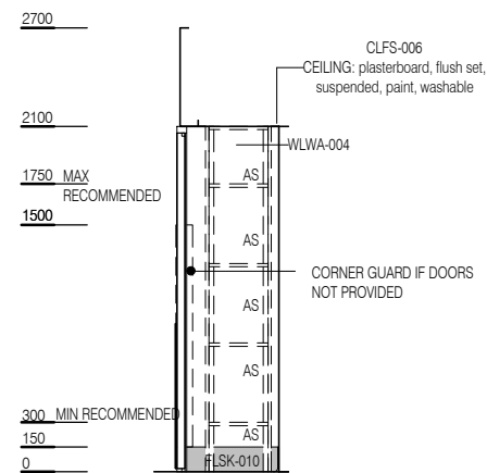
ELEVATION 1
