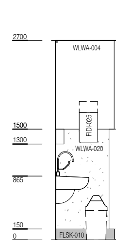
ELEVATION 3
