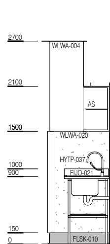
ELEVATION 1
