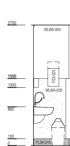
ELEVATION 3
