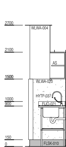
ELEVATION 1
