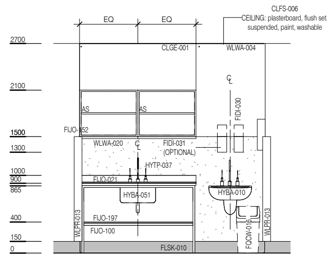
ELEVATION 2
