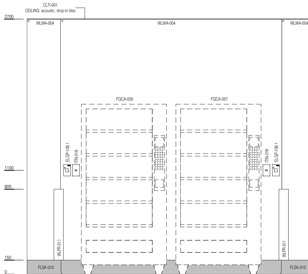
ELEVATION 2
