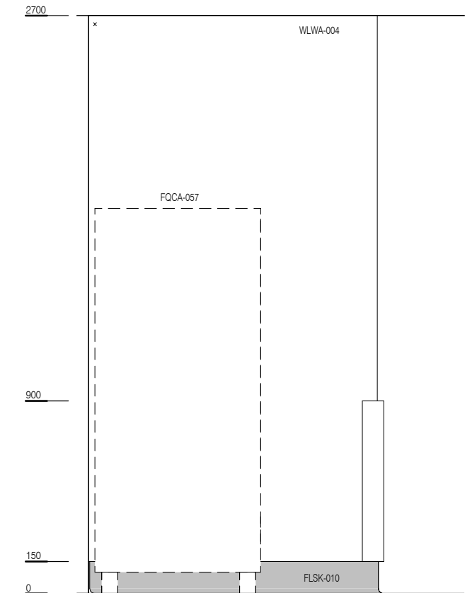
ELEVATION 3
