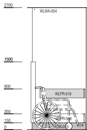
ELEVATION 1
