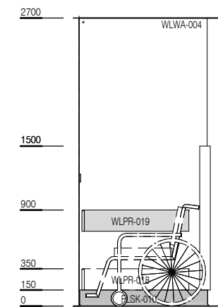
ELEVATION 3
