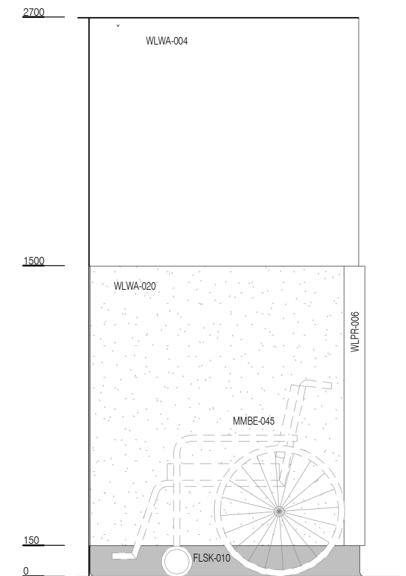
ELEVATION 3
