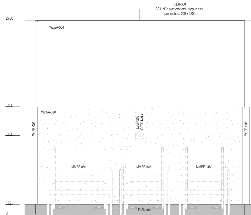
ELEVATION 2
