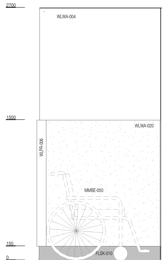
ELEVATION 1
