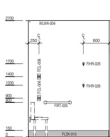
ELEVATION 1
