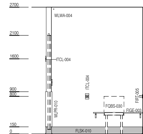
ELEVATION 4
