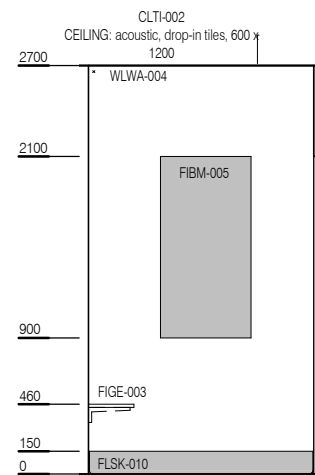
ELEVATION 2
