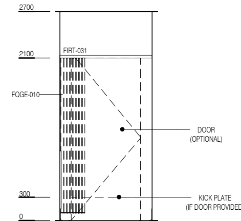
ELEVATION 3
