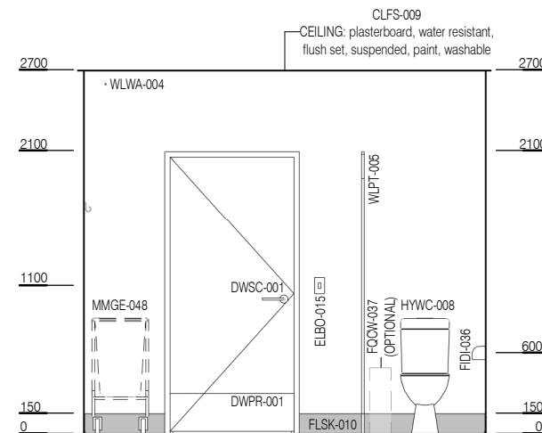
ELEVATION 2
