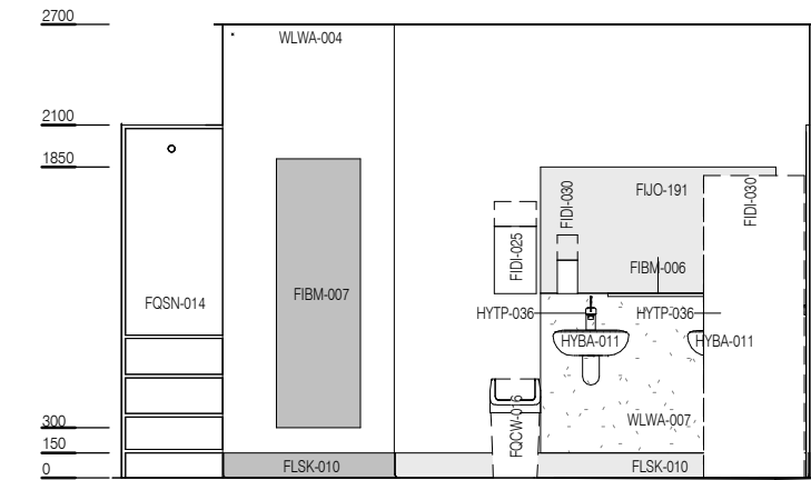
ELEVATION 5
