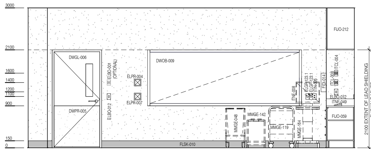
ELEVATION 1
