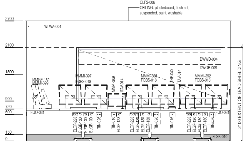
ELEVATION 2
