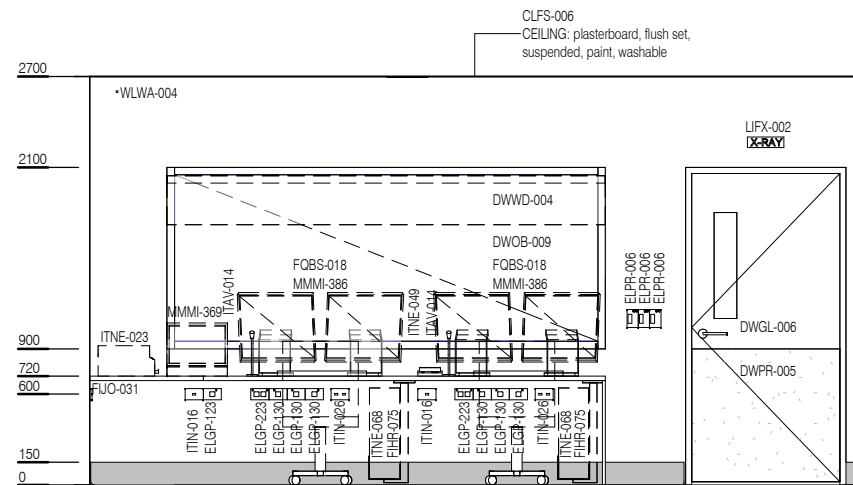
ELEVATION 2
