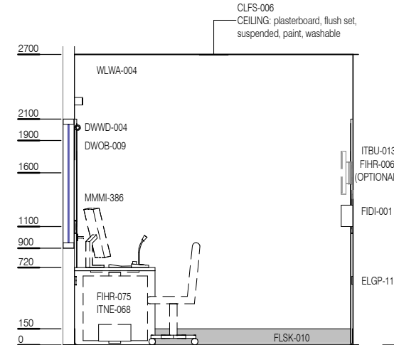
ELEVATION 3
