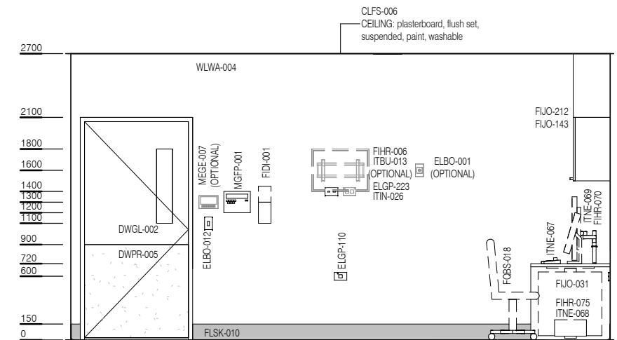
ELEVATION 4
