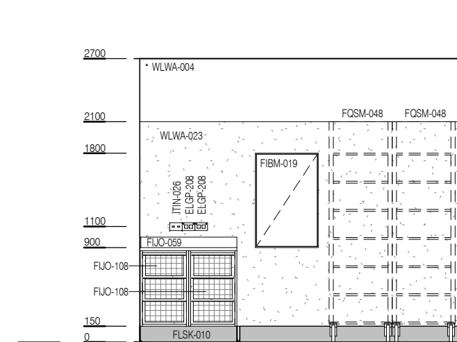
ELEVATION 4
