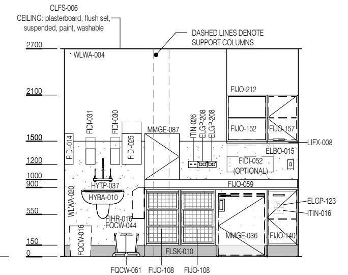
ELEVATION 4
