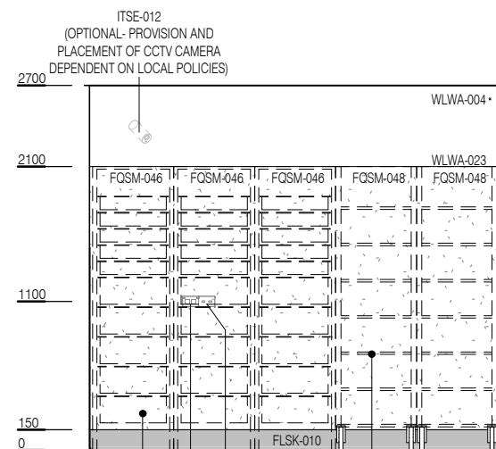
ELEVATION 2
