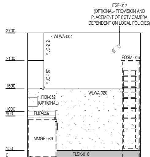
ELEVATION 1
