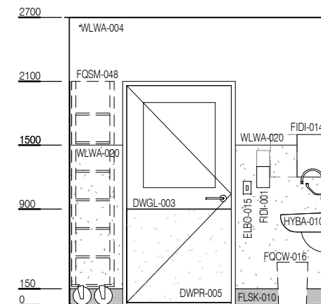
ELEVATION 3
