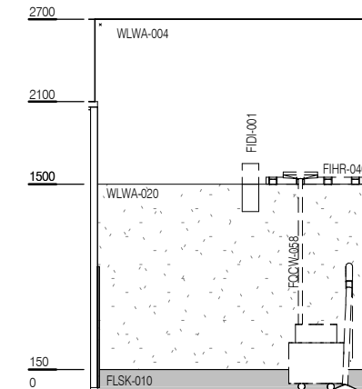
ELEVATION 4
