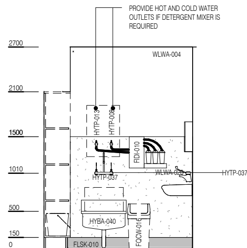
ELEVATION 2
