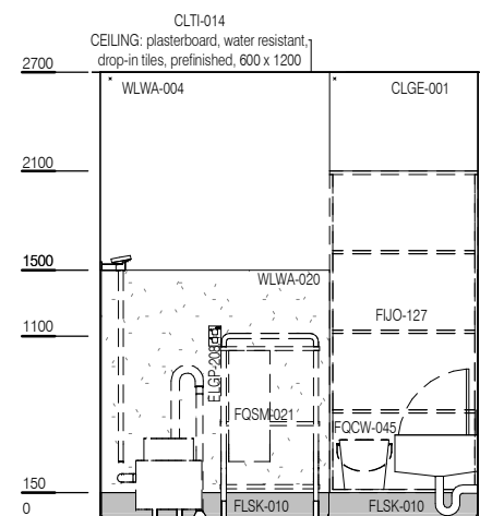
ELEVATION 1
