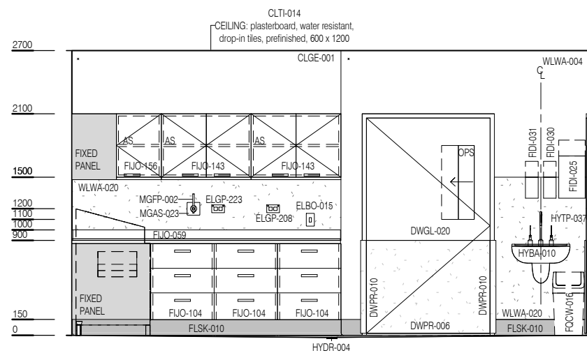
ELEVATION 2
