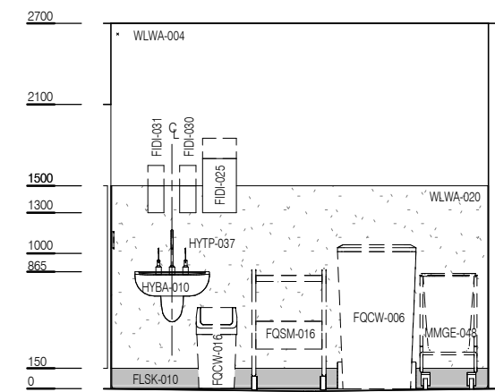
ELEVATION 4
