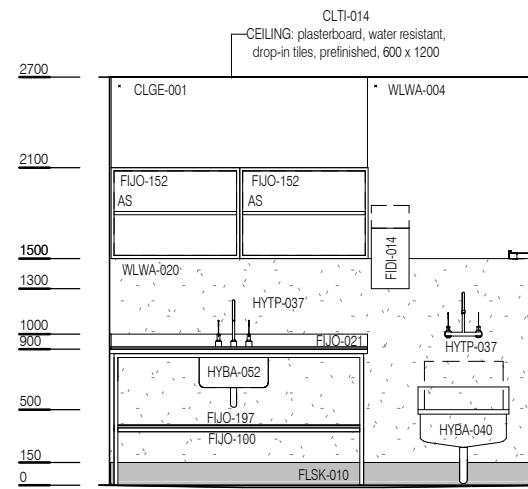
ELEVATION 2
