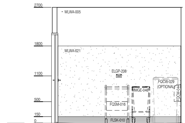
ELEVATION 4
