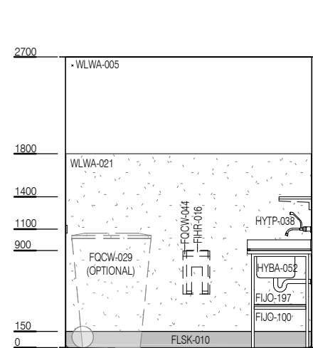
ELEVATION 1
