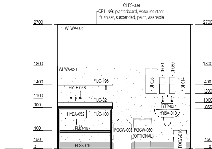
ELEVATION 2
