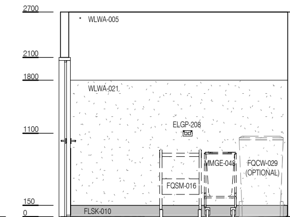
ELEVATION 4
