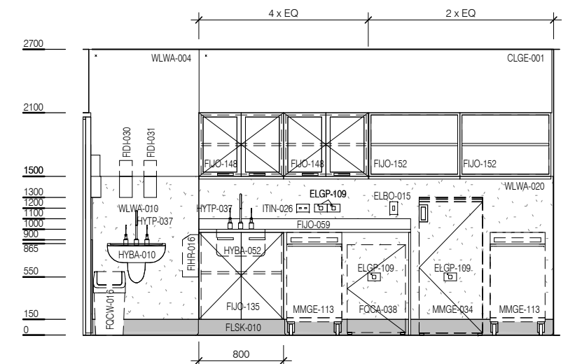
ELEVATION 4
