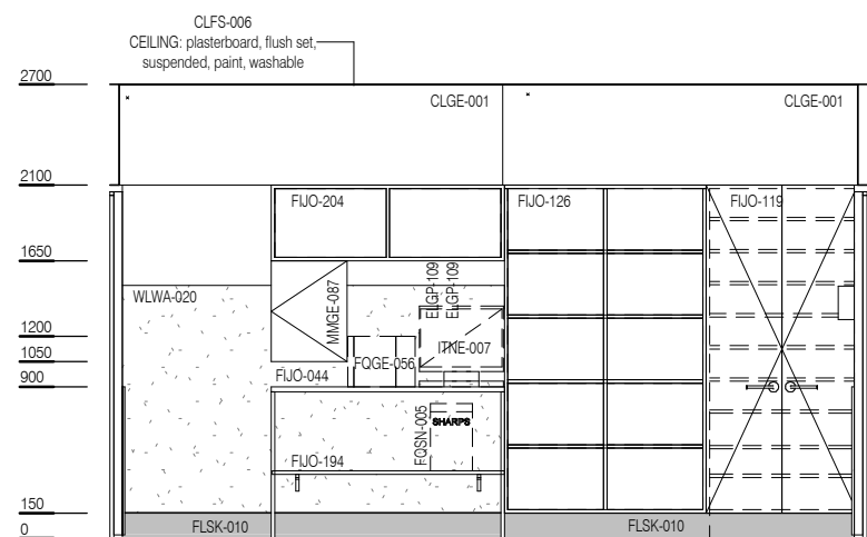
ELEVATION 2
